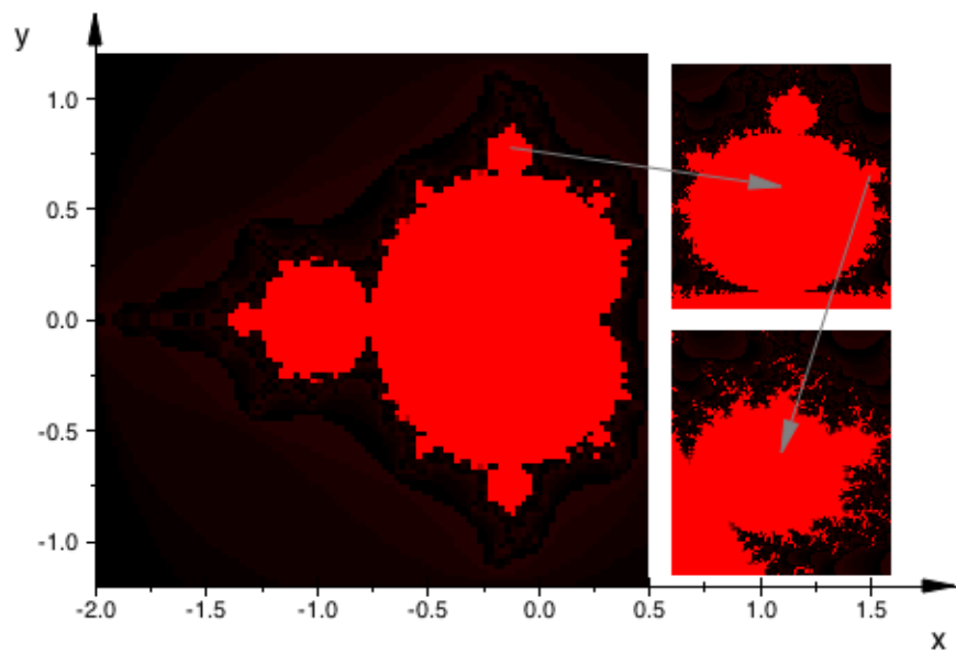
Fig. 13: Mandelbrot Set
