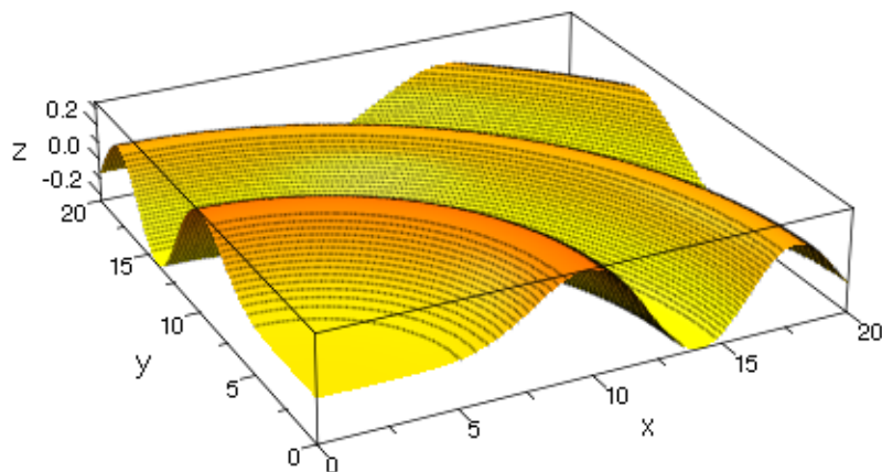
Fig. 18: Bessel Functions
